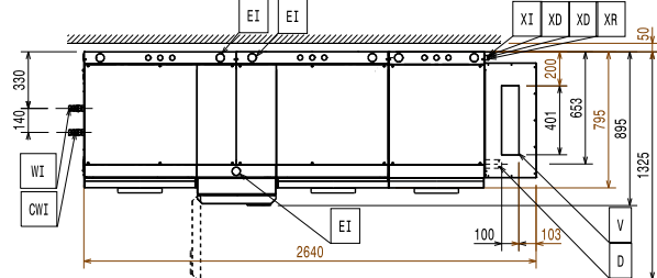
Boven aanzicht
